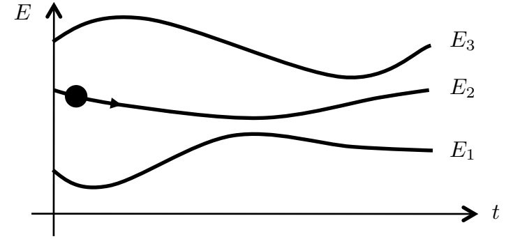
FIGURE 3.1. Variation dans le temps des énergies E_n associées aux états propres |\psi_n\rangle de l'hamiltonien \hat{H}[\lambda] .
