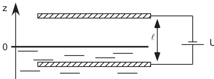
Figure 2: Une tension positive U tend à comprimer les électrons sur la surface de l'hélium, ce qui modifie la position des niveaux d'énergie E_j , j = 1, 2, \dots
